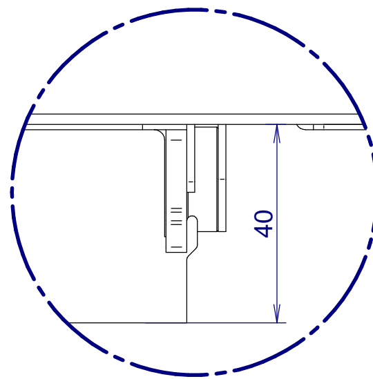
DETAIL A 1:1
